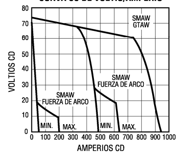
CURVA CC DE VOLTIO/AMPERIO
