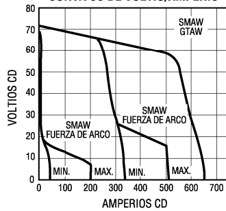
CURVA CC DE VOLTIO/AMPERIO
